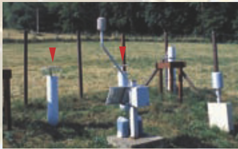
Dispositif de collecte de la pluviosité et des dépôts atmosphériques hors forêt ▼ = collecteur
