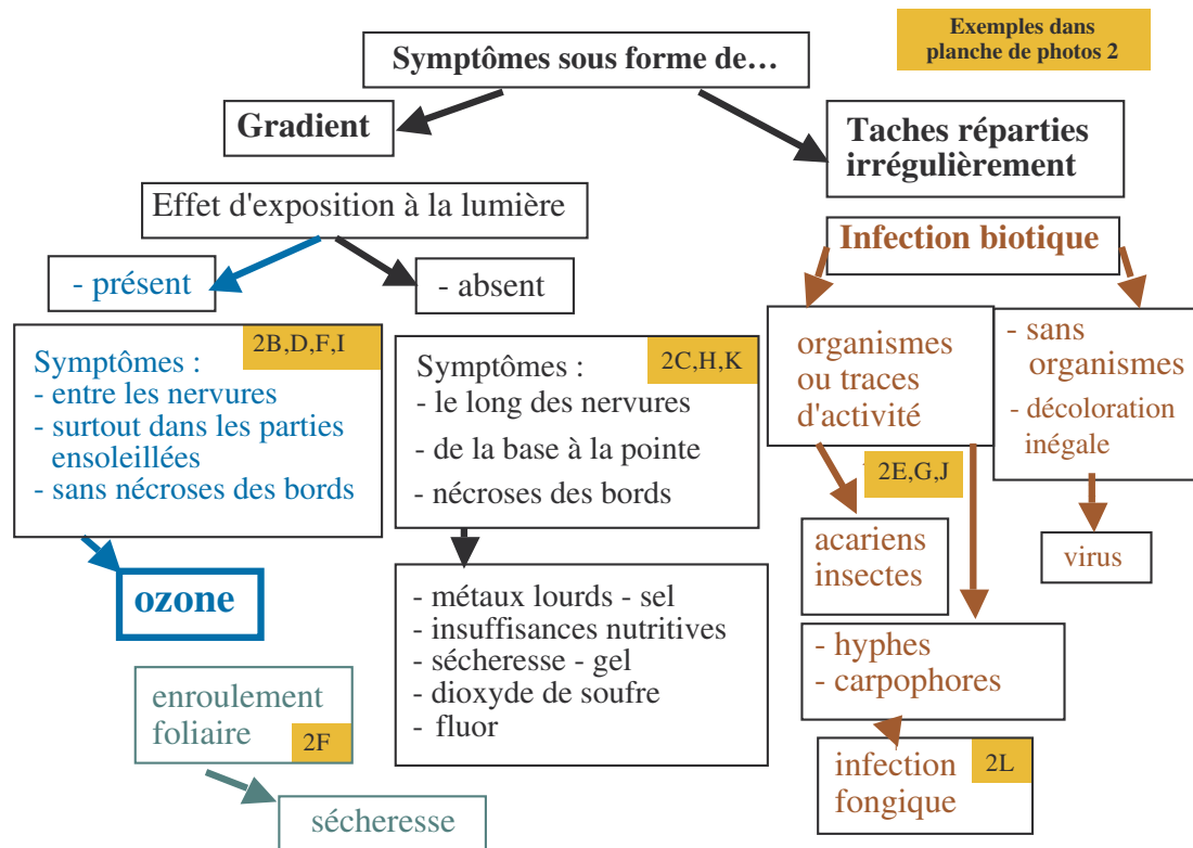
Fig. 1 : critères permettant de différencier, au niveau de la feuille, les symptômes visibles dus à l’ozone de ceux causés par d’autres facteurs de stress (les chiffres et lettres renvoient aux photos de la planche 2)
