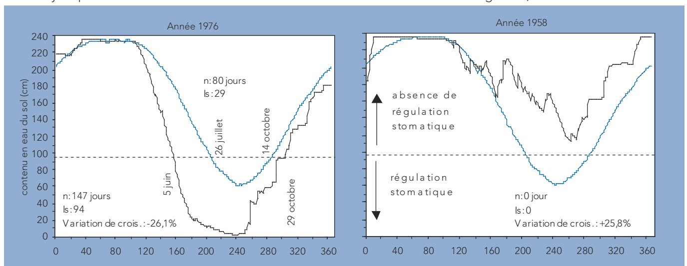
Fig. 2 : évolution (trait noir) de la réserve utile en eau du sol pour l'année sèche 1976 et l'année humide 1958 dans la chênaie sessiliflore de la forêt domaniale de Bercé (72)
