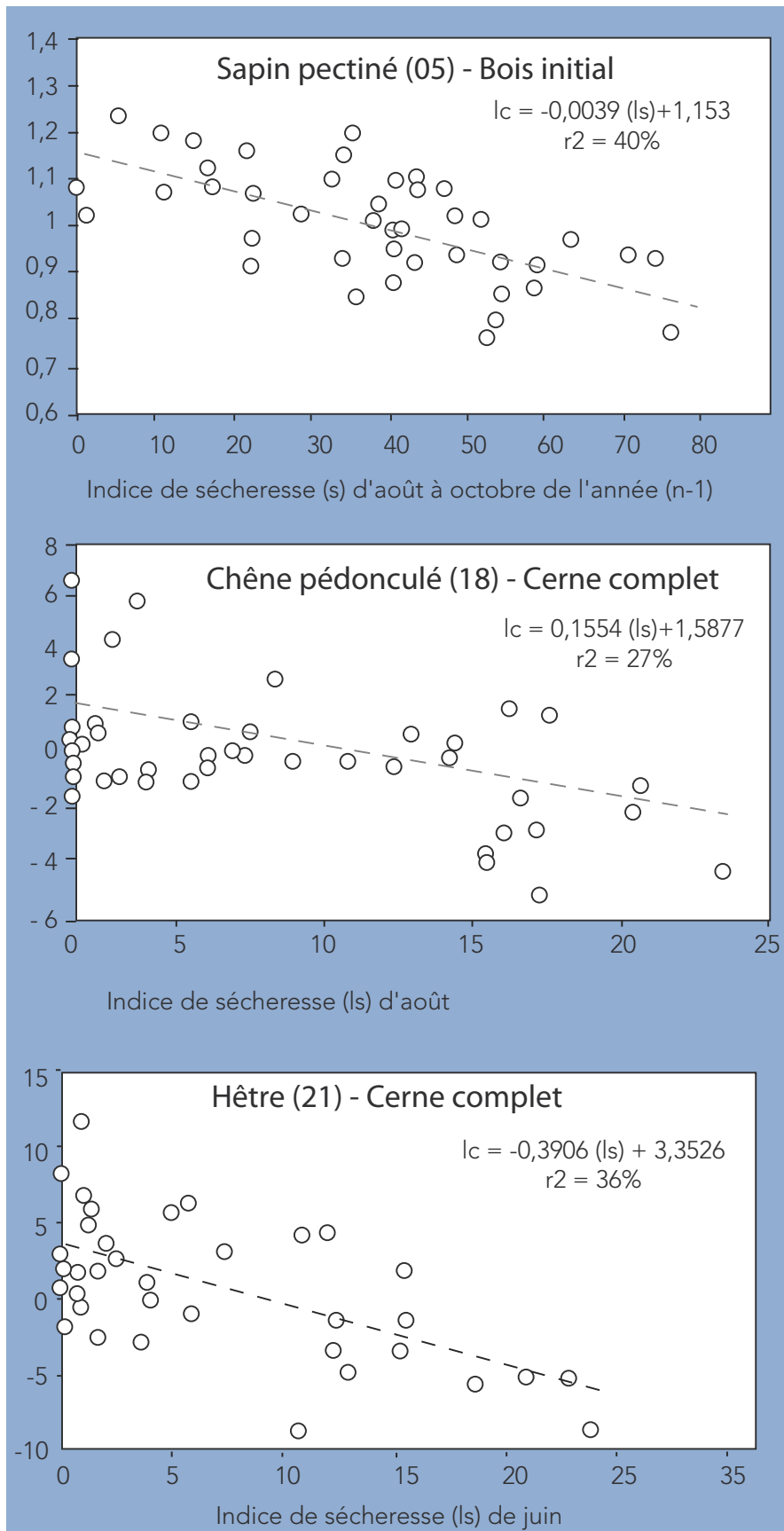
Fig. 3 : exemple de corrélation entre les indices de croissance ( I_c ) et les indices de sécheresse ( I_s ) pour trois peuplements Plus la valeur de I_s est élevée et plus la sécheresse pour la période correspondante est intense.
