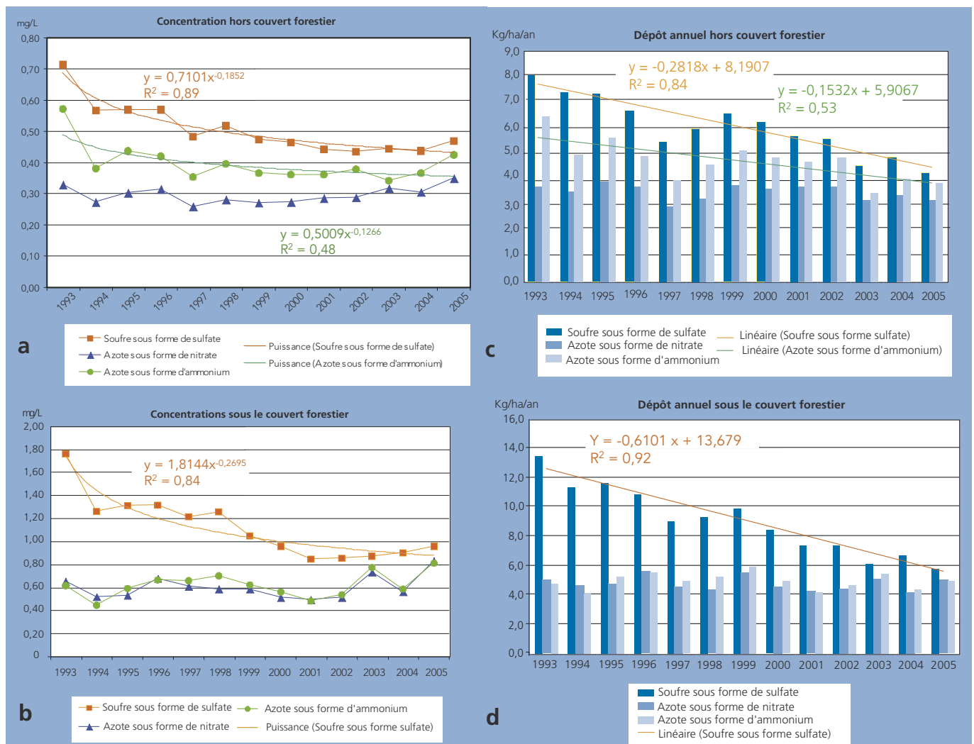
Fig. 4 : évolution de 1993 à 2005 des concentrations moyennes nationales (pondérées par la pluviométrie) (a et b) et des dépôts annuels moyens (c et d) des 27 sites hors et sous couvert forestier pour le soufre (sous forme de sulfate S-SO_4 ), l'azote sous forme de nitrate ( N-NO_3 ) et l'azote sous forme d'ammonium ( N-NH_4 )
