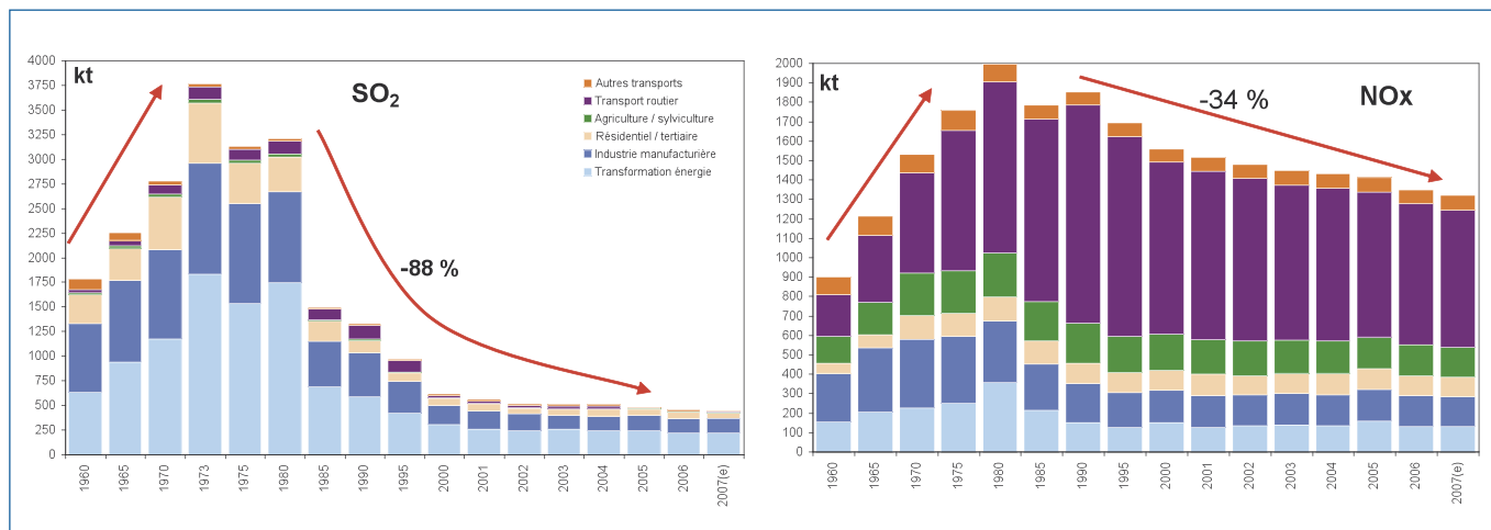
Fig. 1 : évolution des teneurs en SO_2 et en NO_x dans l'atmosphère en France entre 1960 et 2007 (source CITEPA, 2008)
