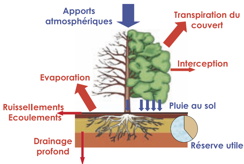
Fig. 1 : le bilan hydrique forestier simplifié
