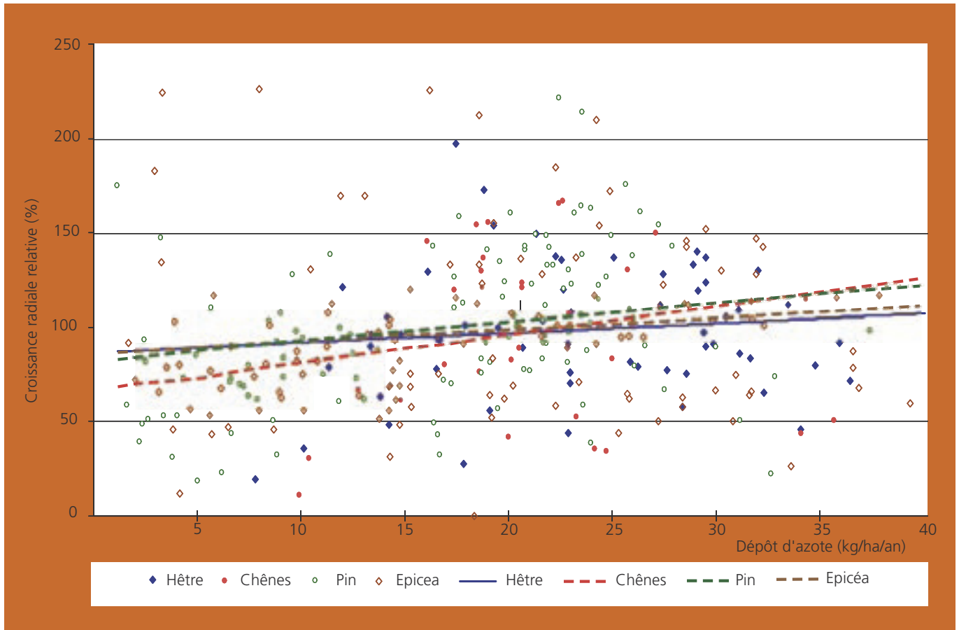
Fig. 6 : relation entre croissance radiale et dépôt d'azote dans le réseau européen de niveau II, dont fait partie RENECOFOR (source : Solberg et al., 2007)
