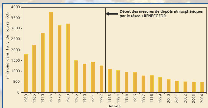
Emissions de dioxyde de soufre dans l'air en France métropolitaine de 1960 à 2004 (source : CITEPA / CORALIE / format SECTEN)
