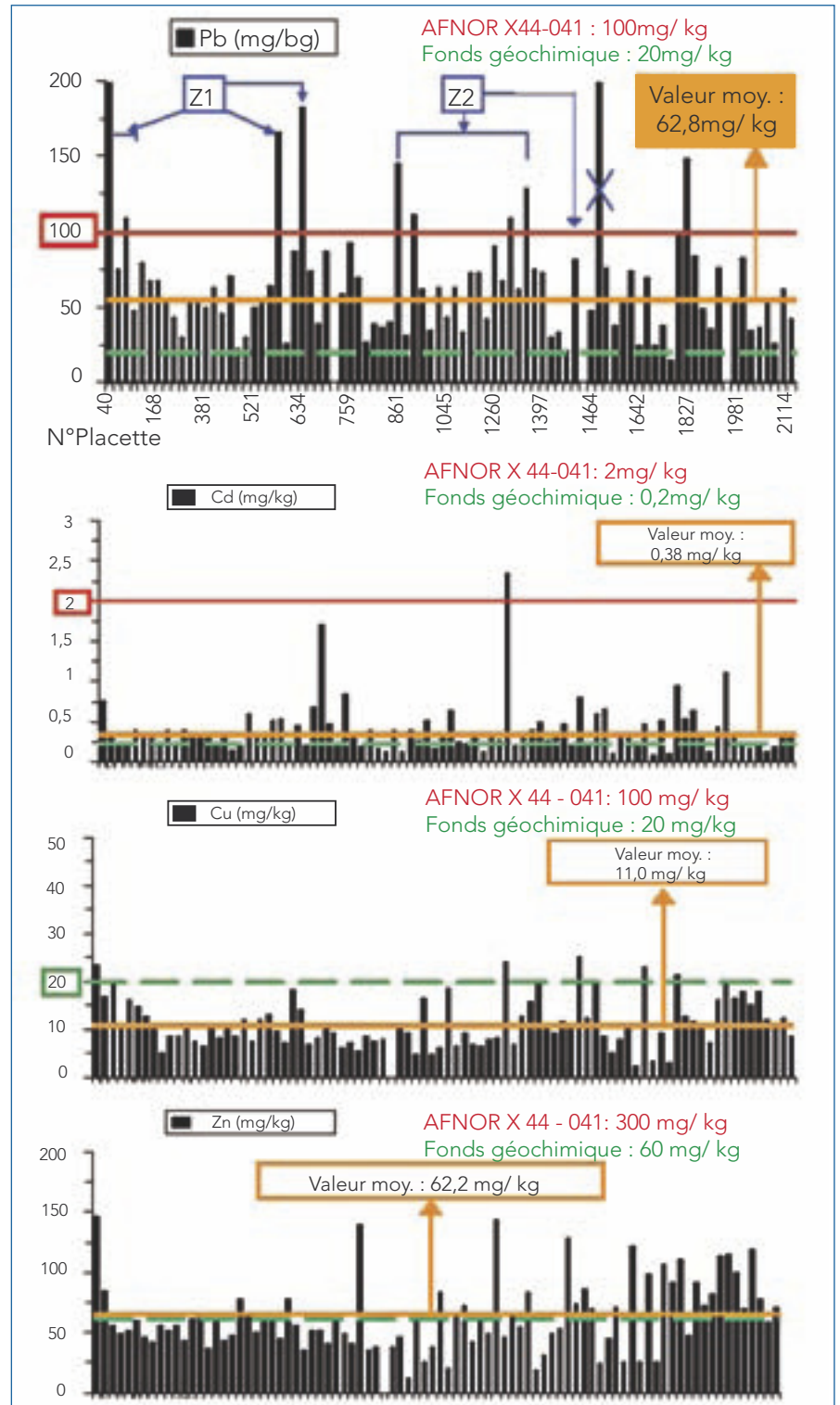
Fig. 2 : comparaison des teneurs en plomb, cadmium, cuivre et zinc dans les horizons holorganiques (OH) des placettes du réseau européen avec le fond géochimique (pointillé vert) et la norme AFNOR (trait rouge) relative aux teneurs en métaux des sols avant épandage des boues d'épuration (Probst et al., 2003)
