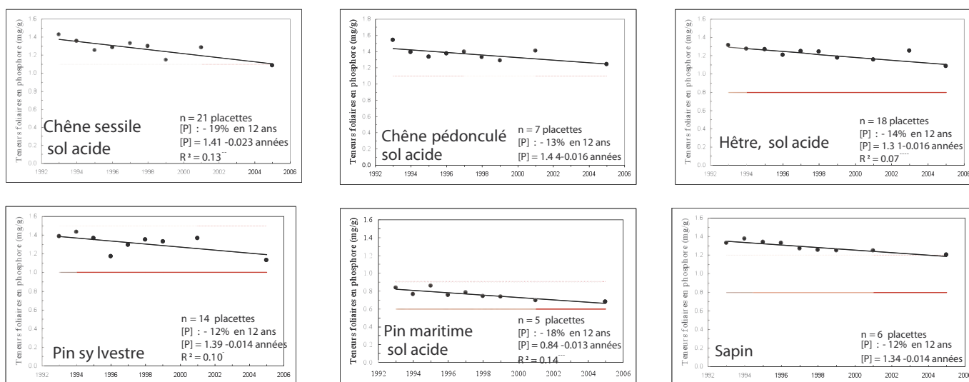
Fig. 2 : évolution des teneurs foliaires en phosphore au cours du temps dans différents groupes de placettes RENECOFOR
