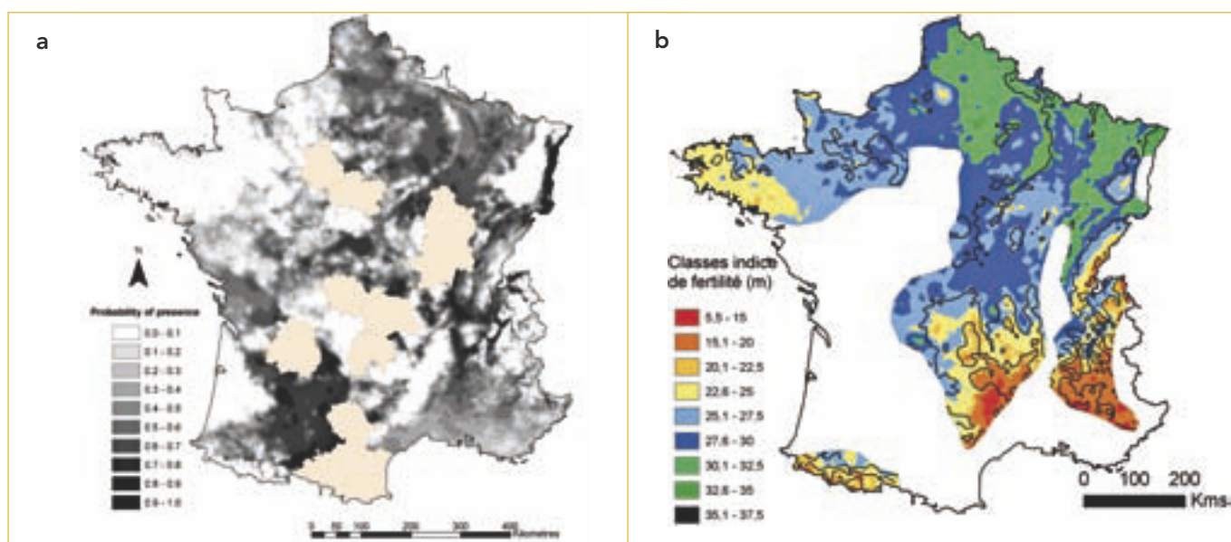
Fig. 1 : cartes de distribution de l'épicéa commun (a) et d'indice de fertilité (hauteur dominante à 100 ans) du hêtre (b) Zones blanches : pas de données suffisantes.
