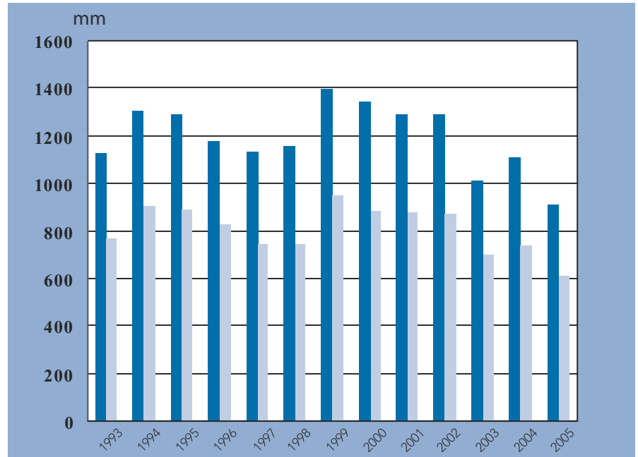
Fig. 5 : pluviosité moyenne annuelle des 27 sites en plein champ (bleu foncé) et sous le couvert forestier (bleu clair) en mm
