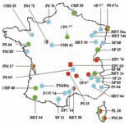
Fig. 2 : les 36 sites RENECOFOR dont les espèces ont été inventoriées par le GIEFS sur les clairières, pour les symptômes d'ozone avec confirmation par le centre de validation de l'institut WSL en Suisse (à l'exception des sites représentés par un carré)
