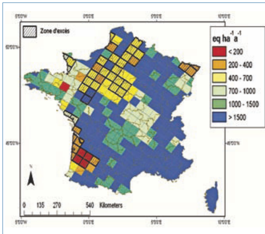
Fig. 5 : carte des charges critiques d'acidité pour les écosystèmes forestiers et zones de dépassement (Probst et al. , 2004)
