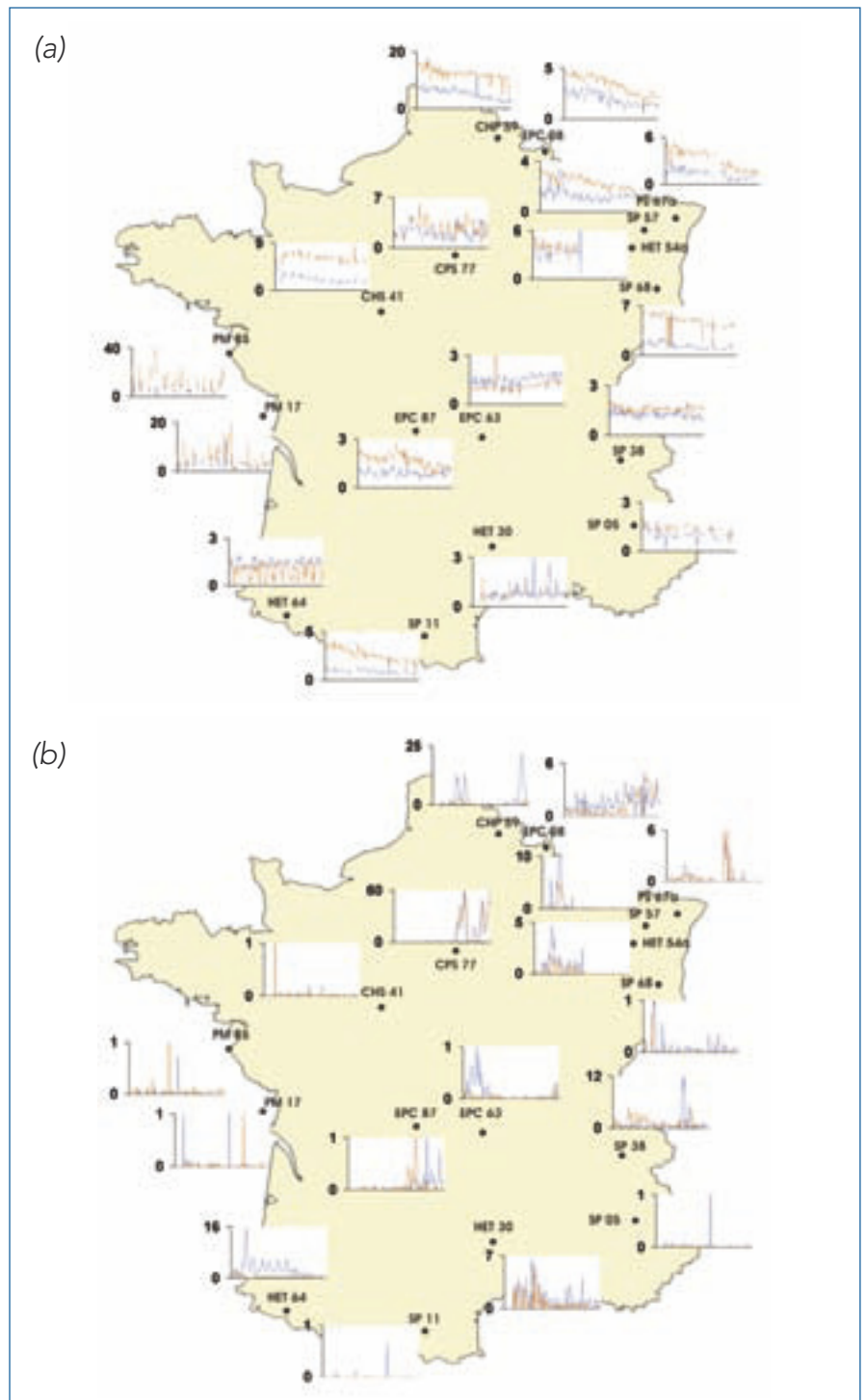
Fig. 1 : concentrations de soufre sous forme de sulfate (a) et concentrations en nitrates (b) des solutions de sol des 17 sites RENECOFOR (en mg/L de soufre et d'azote) de 1994 à 2006 ; en bleu à 20 cm et en orange à 70 cm de profondeur
