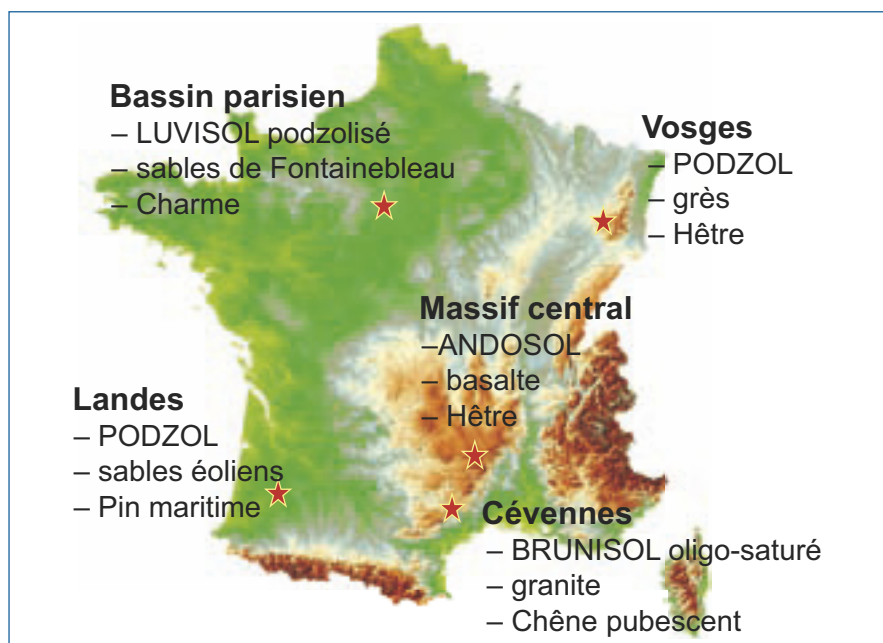
Fig. 2 : exemples d'écosystèmes forestiers de sensibilités variées à l'acidification, pour lesquels les charges critiques d'acidité ont été calculées à partir des mesures faites sur certains sites RENECOFOR
