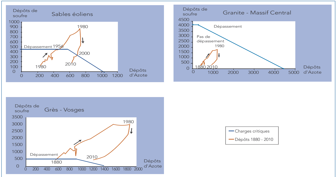
Fig. 6 : évolution des dépôts atmosphériques modélisés en soufre et azote entre 1880 (avant l'ère industrielle) et 2010 (échéance du protocole de Göteborg) et comparaison avec les valeurs de charges critiques (Source : Moncoulon et al., 2007)
