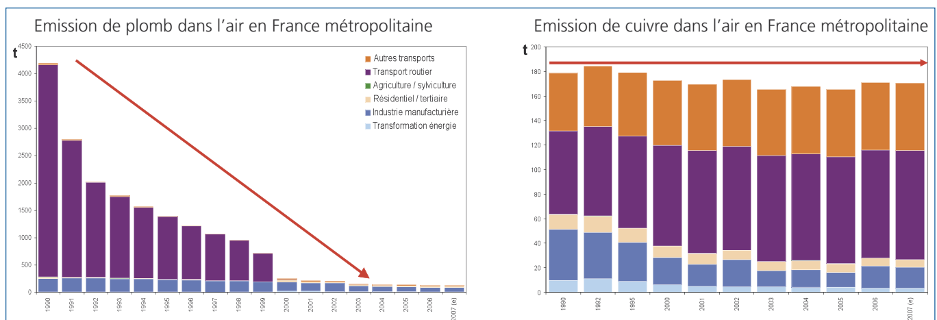
Fig.1 : tendance des émissions atmosphériques de plomb et de cuivre par secteur d'activité en France (source CITEPA, 2008)
